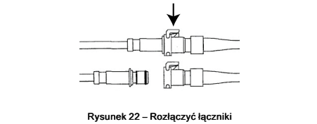
Rysunek Z2 – Rozłączyć łączniki
